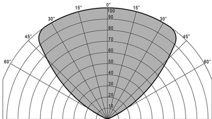
Рисунок 5 - Зависимость дальности обнаружения очага пламени от его углового положения в поле зрения извещателя в процентах от максимального значения
